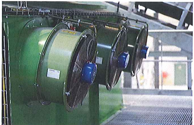
Wyposażenie sortowni
