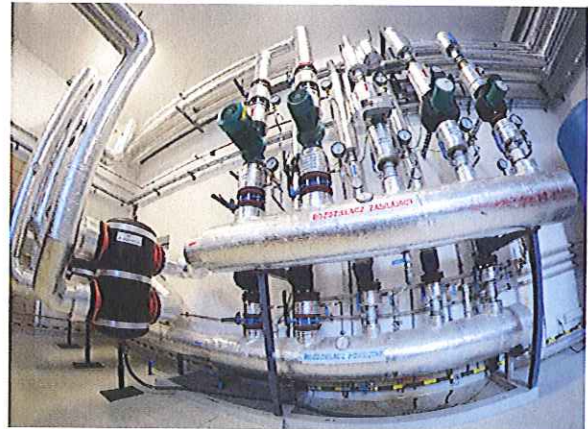
Bioelektrownia – Kotłownia
